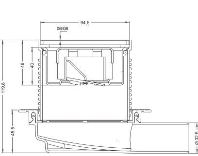
Ø 32 YAN ÇIKIŞ
